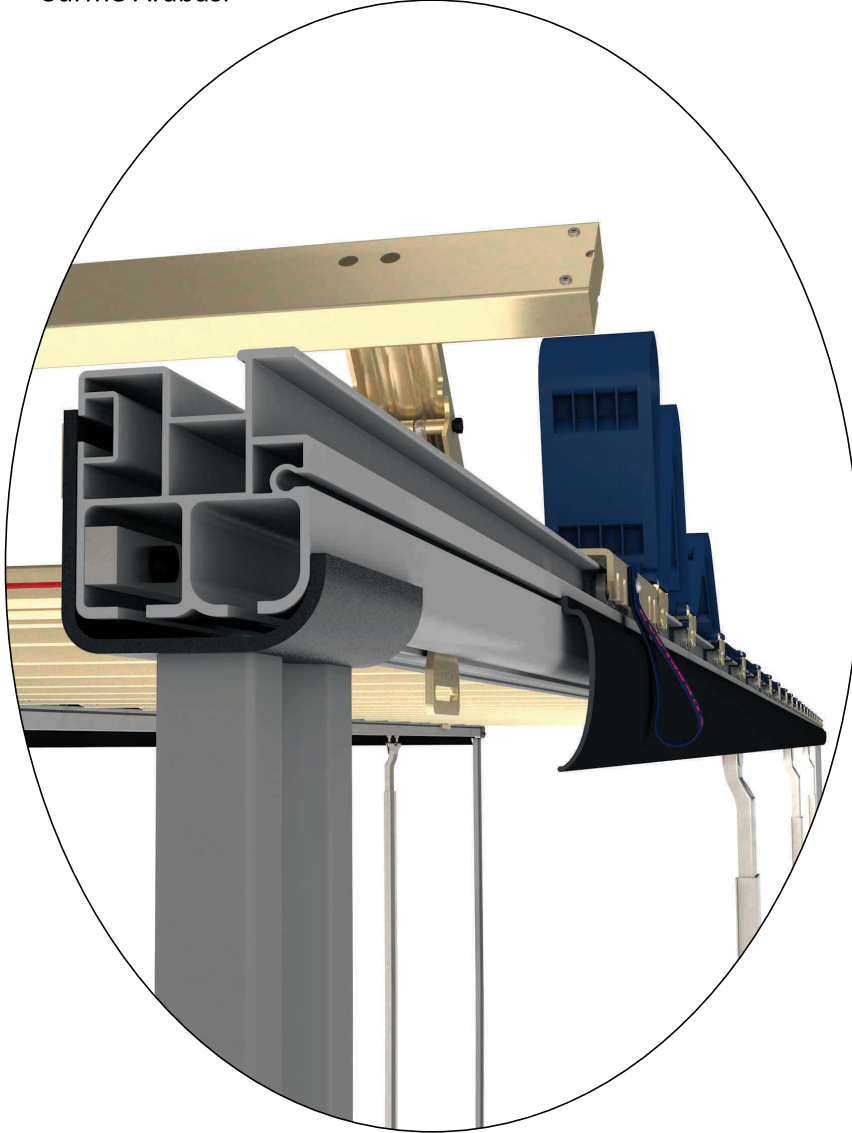
Z Tipi Kayar Baba Makarası
